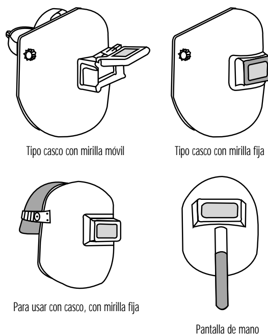
Figura 31.4 • Protectores para soldadura.
